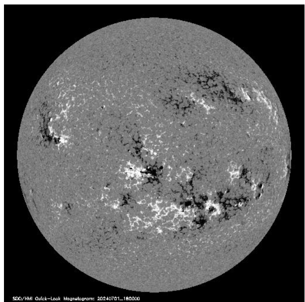
Bild 6 Magnetfeld-Flecken
