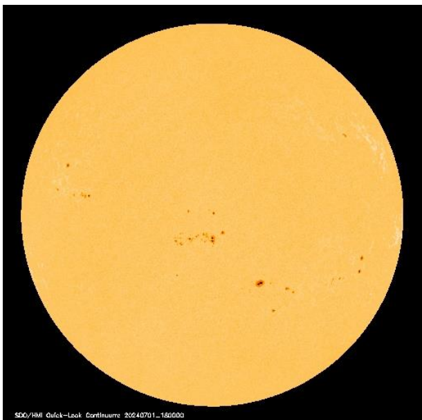
Bild 5 visuelle Sonnenflecken
