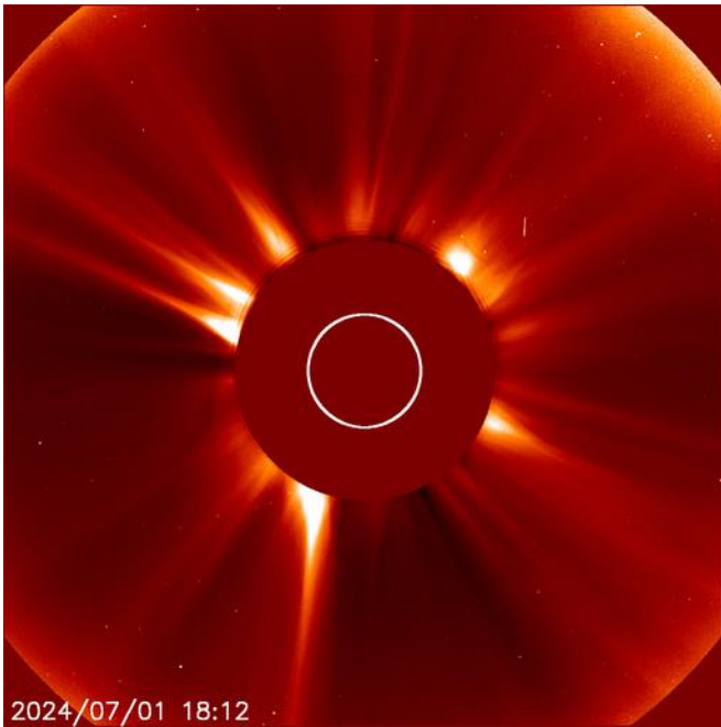
Bild 7 C2- Korona-Aufnahme
