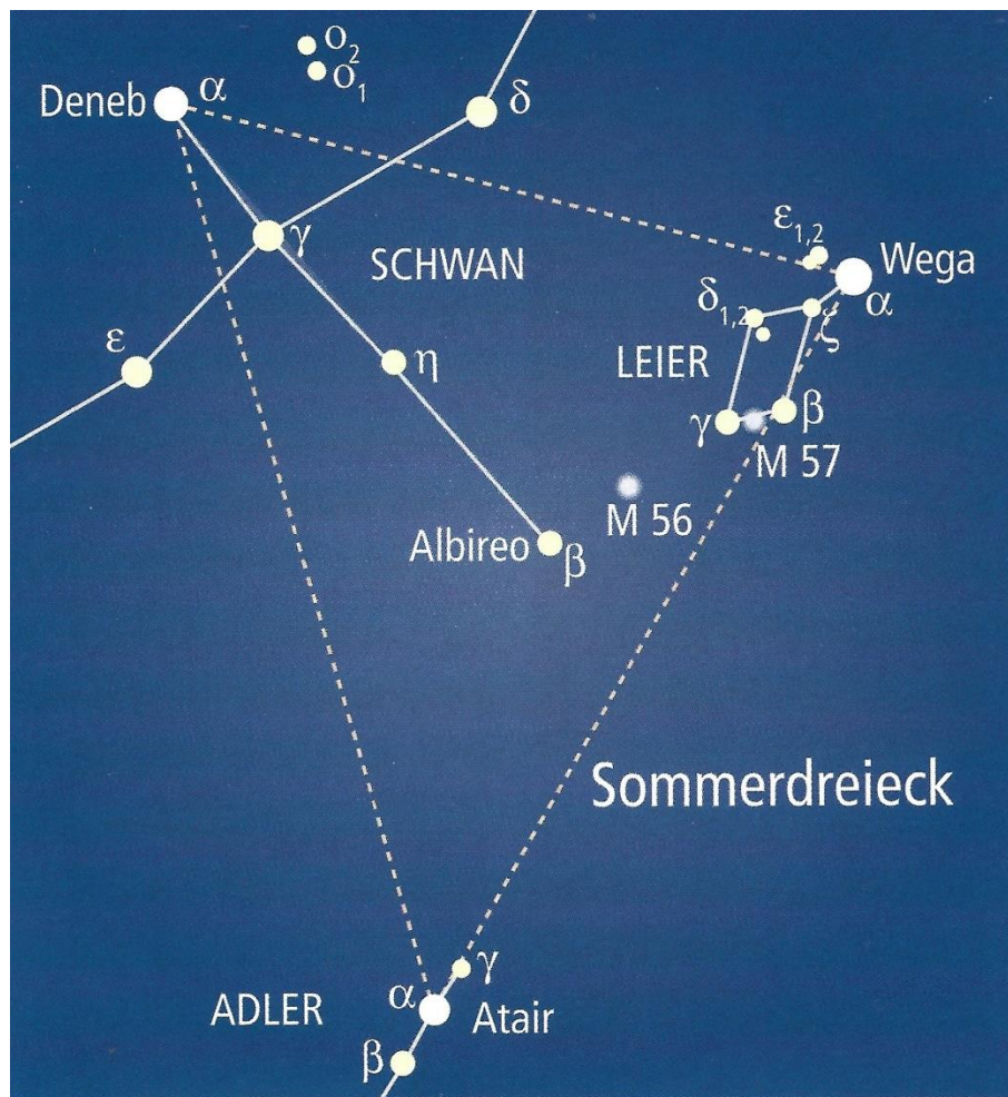
Bild 3 Sommerdreieck
